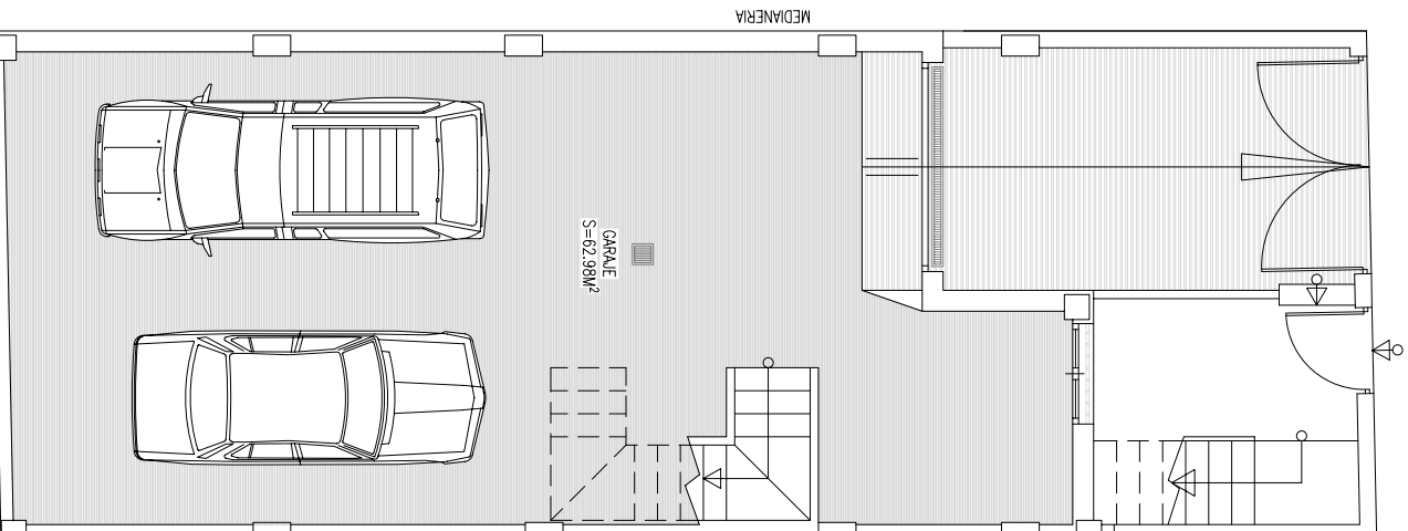
PLANTA SEMISOTANO
