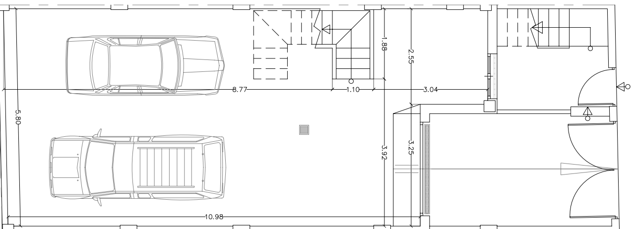
PLANTA SEMISOTANO
