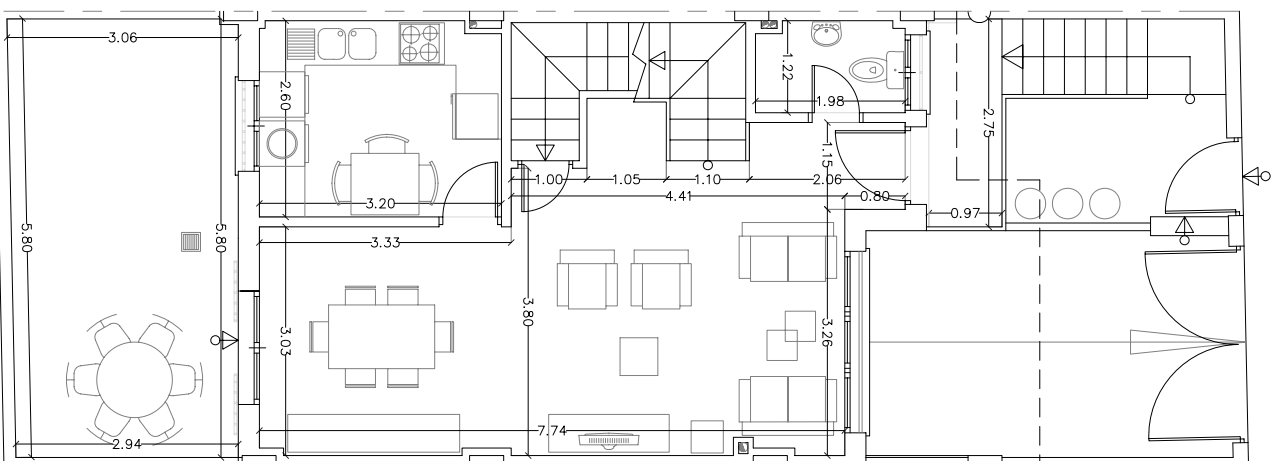
PLANTA BAJA
