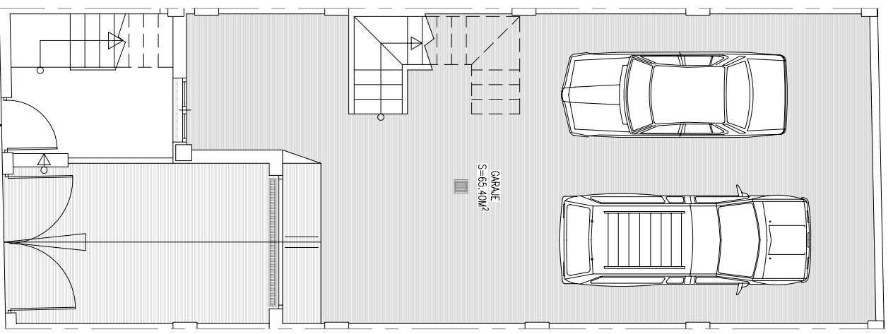
PLANTA SEMISOTANO
